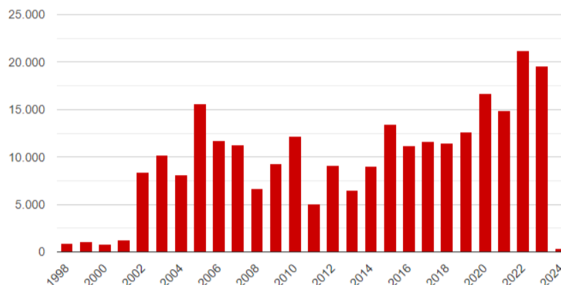
Gráfico 1 - Série histórica do total de focos ativos detectados no estado do Amazonas pelo satélite de referência, no período de 1998 até 26/Mai.
